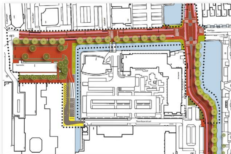
Ontwerp centrumring met het betreffende werkgebied
